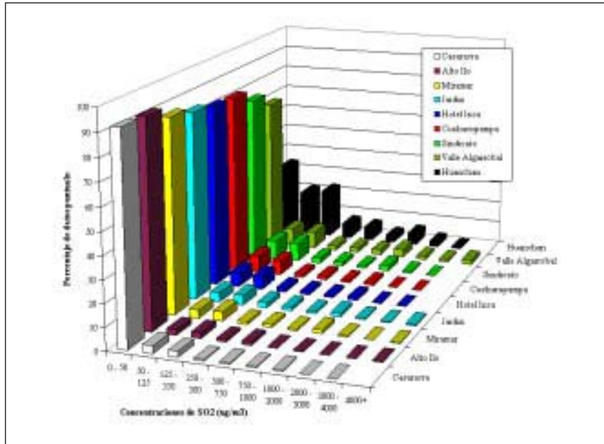
Gráfico 10. Histogramas de las estaciones de monitoreo de La Oroya (Huanchán, Sindicato, Cushurupampa, Hotel Inca, Casaraca) e Ilo (Valle Algarrobal, Jardín, Miramar, Alto Ilo) mostrando el porcentaje de muestras de la calidad de aire que están dentro de los rangos de \text{SO}_2 especificados.
