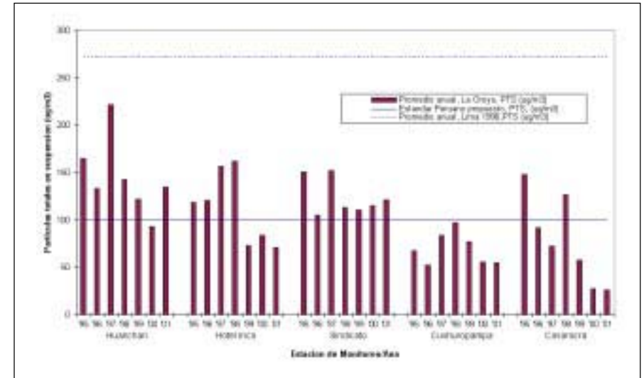
Gráfico 9. Niveles de Material Suspendido Total en las estaciones de monitoreo de La Oroya comparadas con la propuesta de estándares de calidad de aire propuestos por DIGESA (1998). Información que no estaba disponible y por lo tanto no ha sido incluida en los promedios anuales: todas las estaciones de monitoreo 7-12/96, y posteriores a 11/01; Huanchán 9-12/99, 1-3/00; Sindicato 6/00; Cushuropampa 9-12/99, 1-3/00; Casaracra 9-12/99, 1-2/00.
