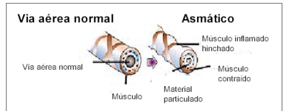
Figura A1-1: Diferencias entre vías aéreas normales y asmáticas. Figura adaptada de Healthy Way: the Health Journal
