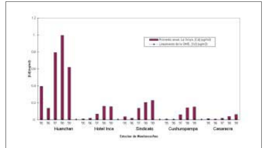
Gráfico 6. Promedio anual de las concentraciones de cadmio medido en las estaciones de monitoreo de la fundición de La Oroya, comparado con el lineamiento de la OMS (0.005 µg/m 3 ).
